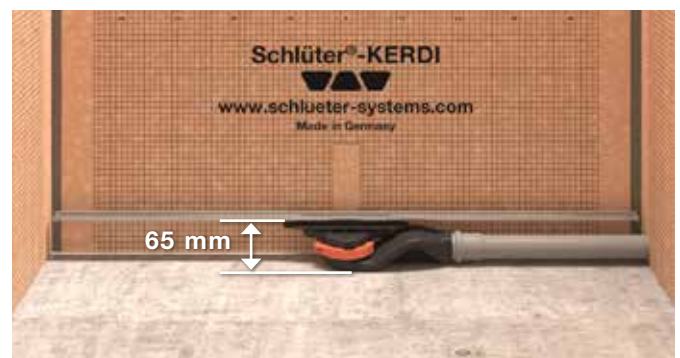
Lage inbouwhoogte: 65 mm
